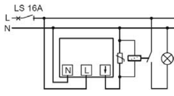
Zapojení se zhásecím RC členem a relé (RC člen se doporučuje při spínání indukčních zátěží (transformátory, cívky stykačů a relé apod.)
